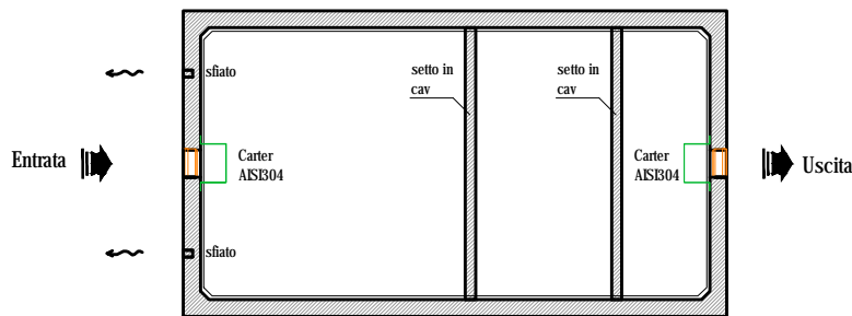
PIANTA VASCA
