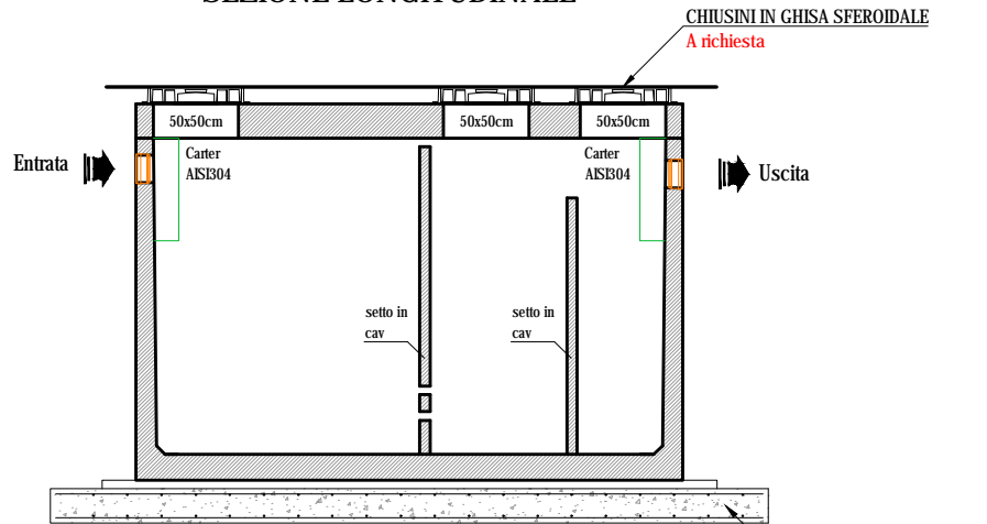
SEZIONE LONGITUDINALE
